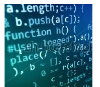
Algorithmische Verfahren
